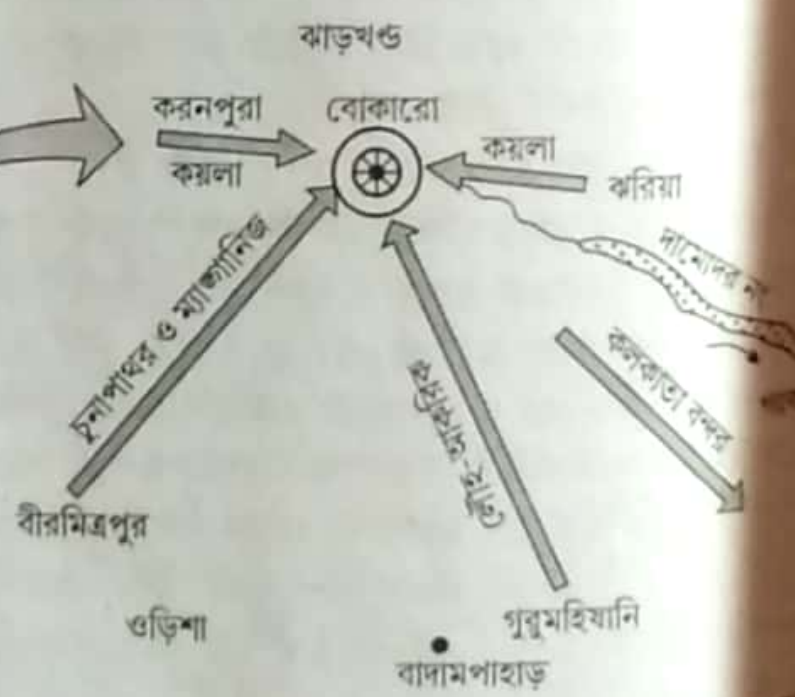
চিত্র : বোকারো লৌহ-ইস্পাত কেন্দ্র
